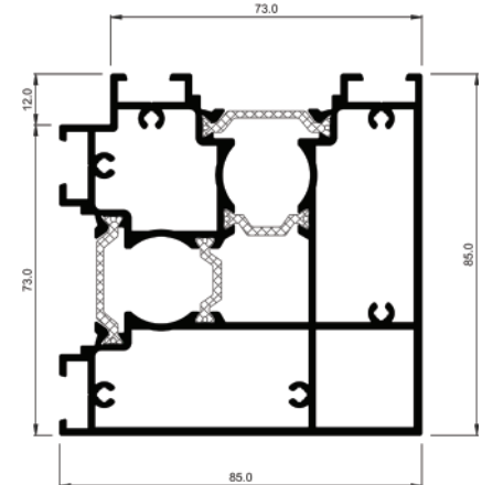
COR-3760 90° corner
